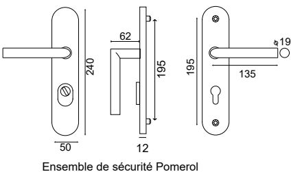
Ensemble de sécurité Pomerol
