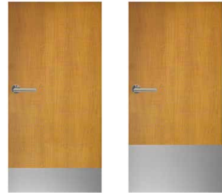
1.Hauteur 250mm
