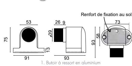
1. Butoir à ressort en aluminium
