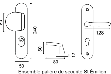
Ensemble palière de sécurité St Émilion
