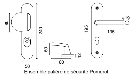
Ensemble palière de sécurité Pomerol
