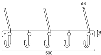
2. Patère fil sur lisse
