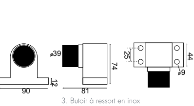
3. Butoir à ressort en inox
