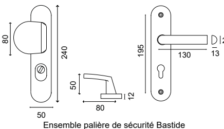
Ensemble palière de sécurité Bastide
