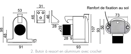
2. Butoir à ressort en aluminium avec crochet
