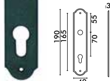
2. Plaque classique PVC
