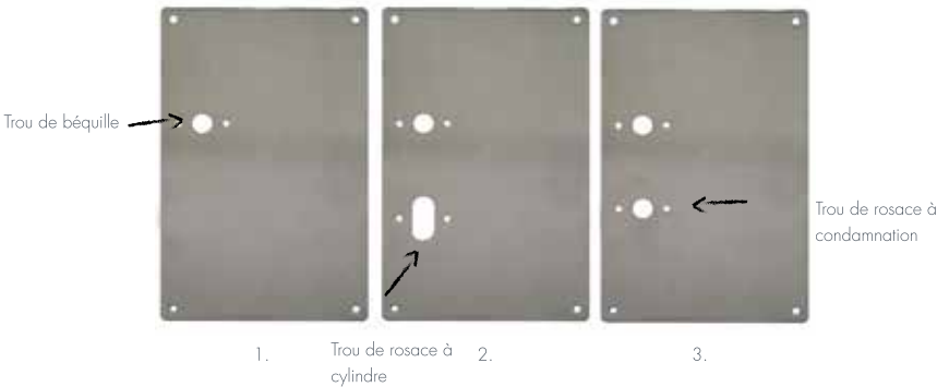
Plaquette universelle présentée avec notre ensemble St Émilien et rosace cylindre à commander séparément
