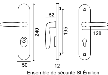
Ensemble de sécurité St Émilion
