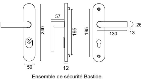
Ensemble de sécurité Bastide
